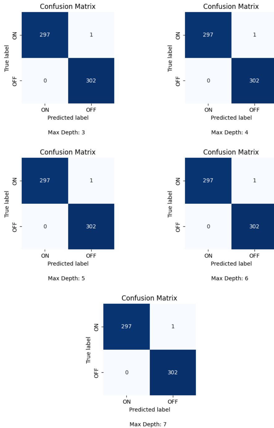
Gambar 5.21 Confusion Matrix pada Variasi Max Depth
