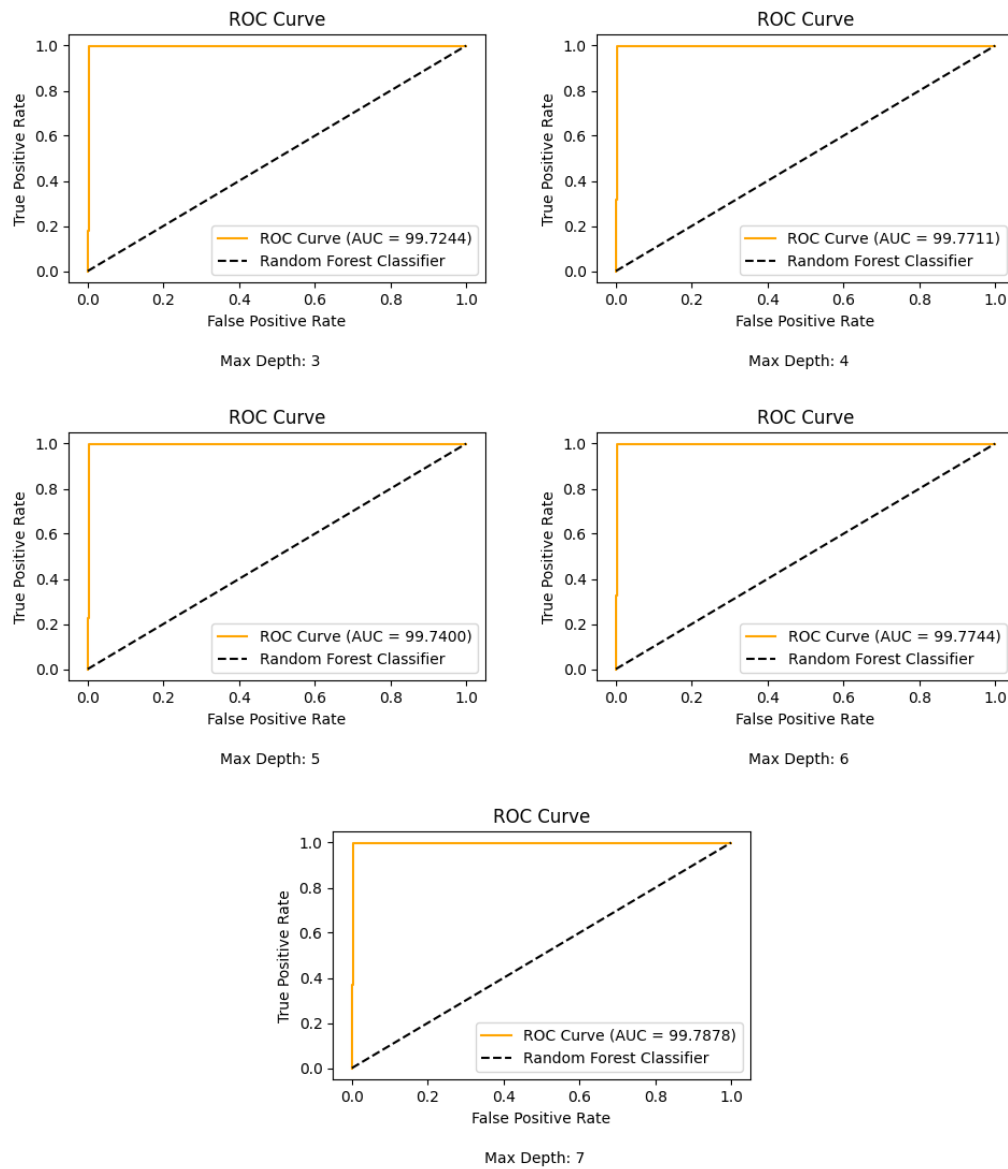
Gambar 5.20 Kurva ROC-AUC pada Variasi Max Depth
